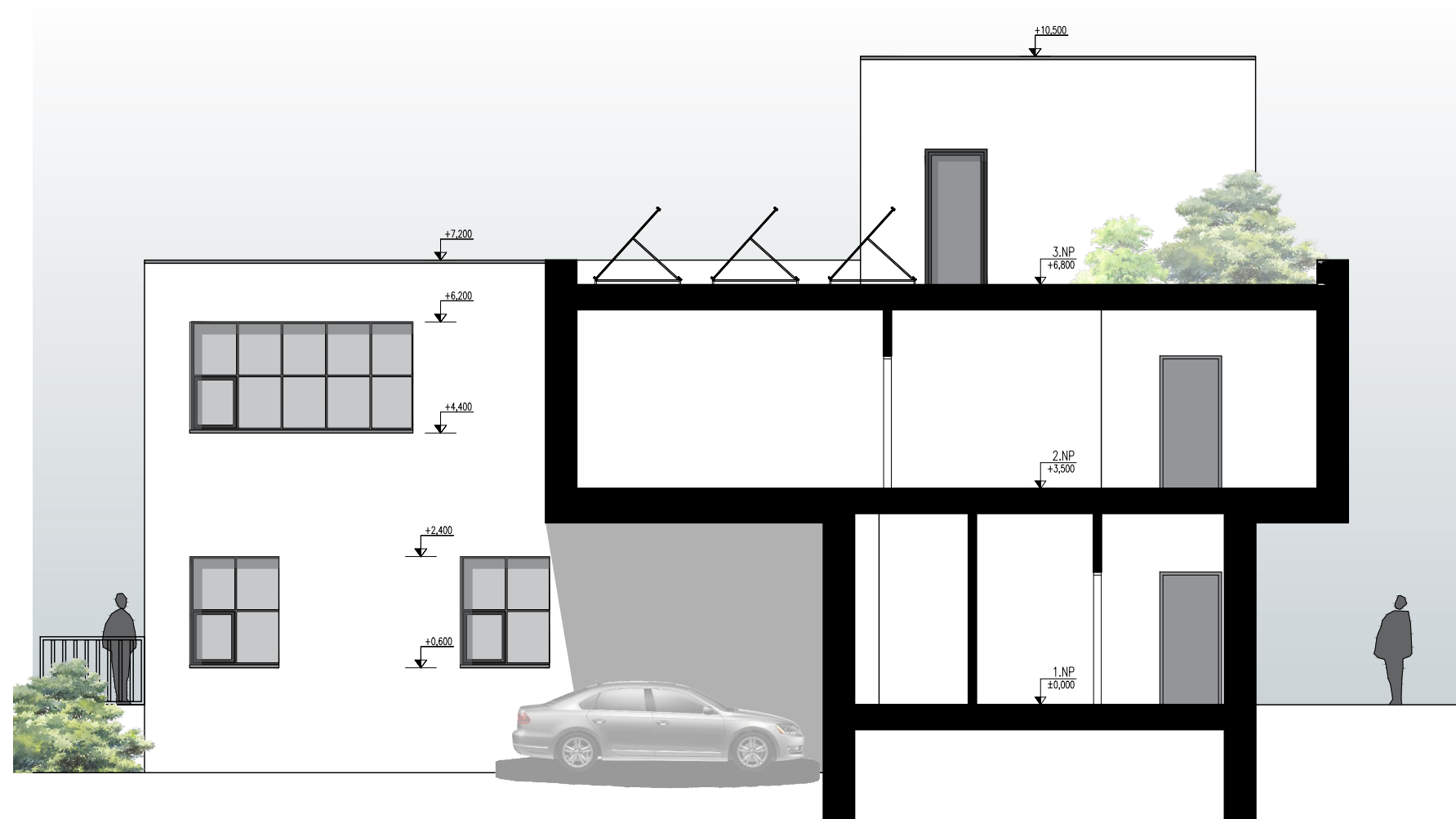
ŘEZ A-A'
