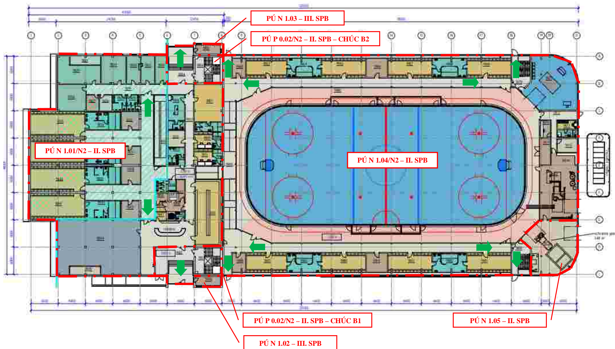
POŽÁRNÍ VÝKRES - PŮDORYS 1.NP - STUDIE
